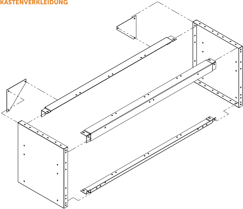
SCHEMA DI MONTAGGIO COPRIPASSARUOTA APERTO ASSEMBLY DRAWING OPEN WHEELHOUSE COVER BAUSCHEMA OFFENE RADKASTENVERKLEIDUNG
